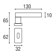
Cod. 140 CS 35 RQ Maniglia per finestra DK Window handle DK
