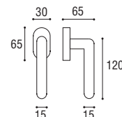
Cod. 152 CS 29 Cremonese EZ Window handle EZ
