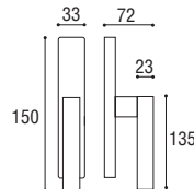
Cod. 174 CS 59 RQ Cremonese EZ Window handle EZ
