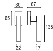
Cod. 180 CS 59 RQ Cremonese EZ Window handle EZ
