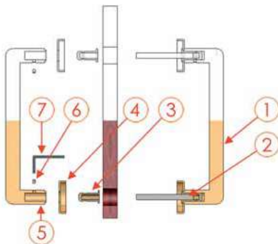
Sezione del montaggio dei maniglioni accoppiati.
