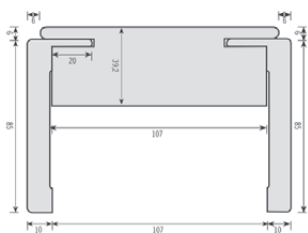
Particolare TELAIO con RINGROSSO "A"
