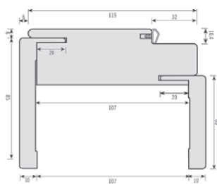
Particolare PASSATA e con ingresso "A"
