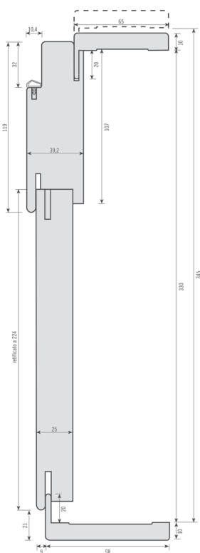
Particolare TELAIO con RINGROSSO "B"
