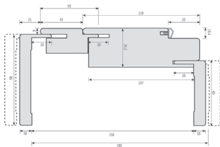
Particolare TELAIO con RINGROSSO "B"
